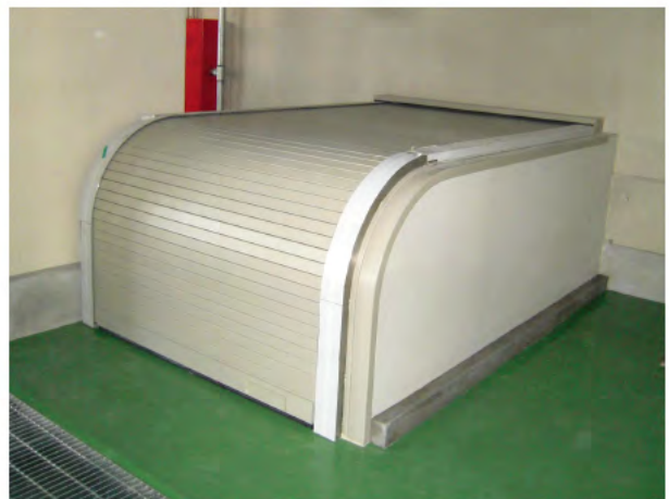
W1,600×H1,200×D6,200 スチール製、電動式、BOX型、 t=1.6 p=75、防火防煙仕様、非常電源バッテリー付き
