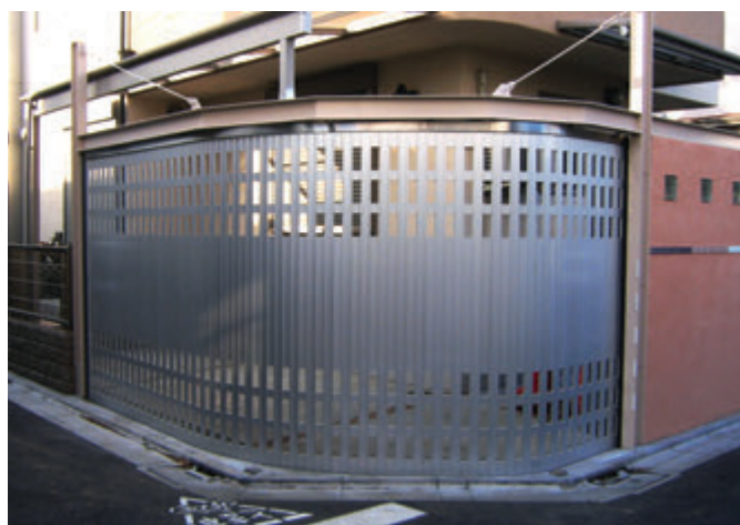
約・W5,200×H2,300 アルミ製（シルバー）手動式、片引き仕様、BOX型、曲げR=300×2カ所
