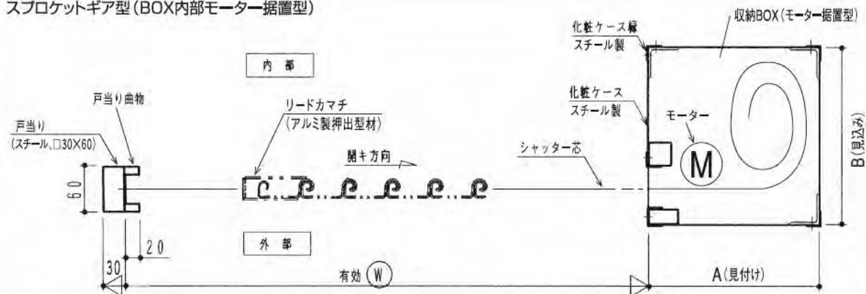
■平面納まり図 (標準仕様):電動式
