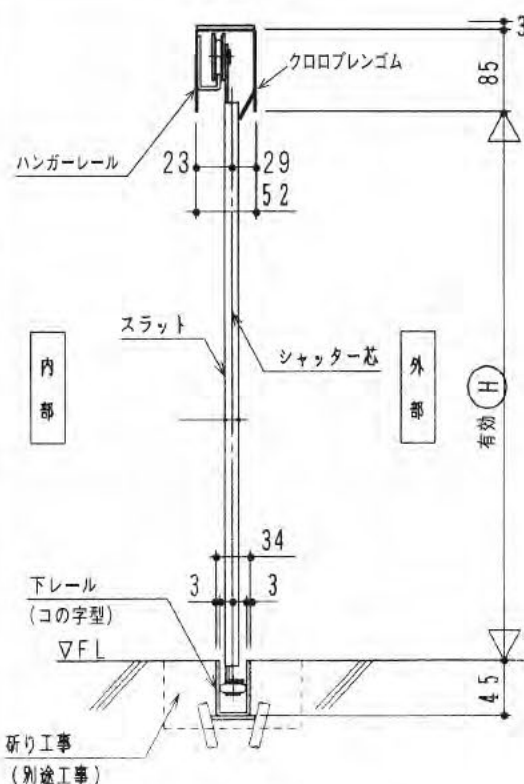
■断面納まり図 (標準仕様)
