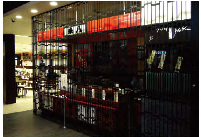
W6,000×H3,000 アルミ製パイプ( 電解着色:ブラック )、片引き仕様、曲げR=600
