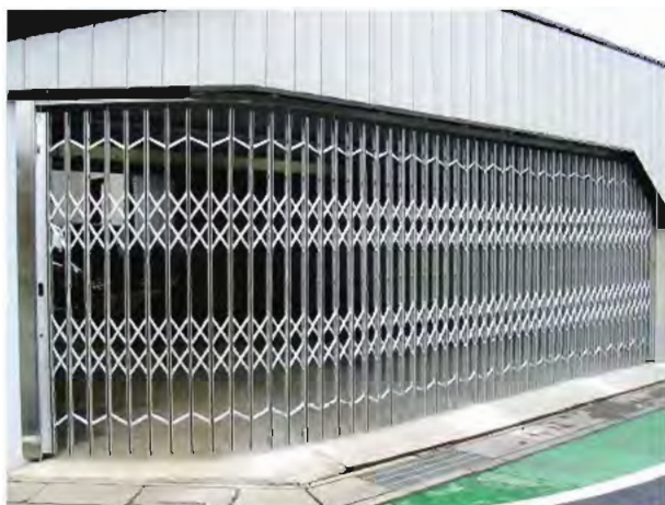
W8,200×H2,300 アルミ製(シルバー) 片引き仕様 フリー型、曲げR=900、下レールなし
